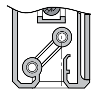
geschraubte Zugentlastung
